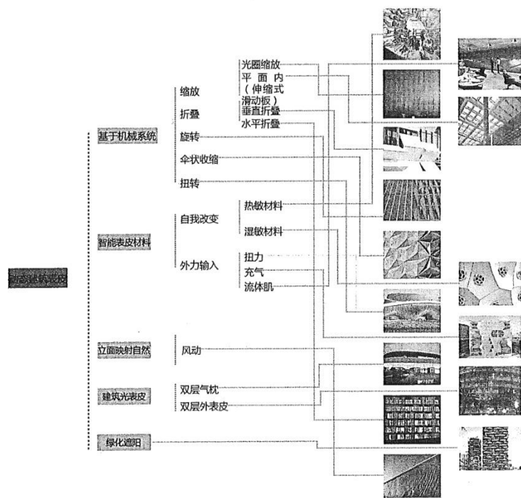
图1 动态表皮可变单元结构设计原理
