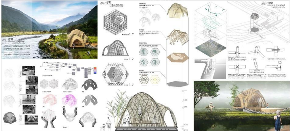
《竹穹》作品图纸
